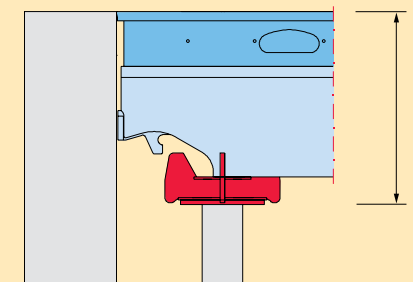
Configurazione della cassaforma con testa d'appoggio non adiacente alla parete.
