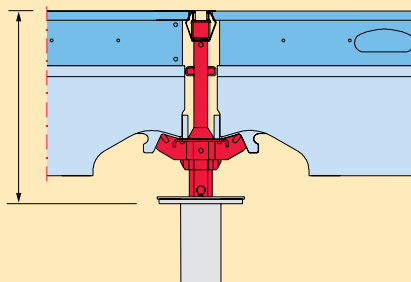
Configurazione della cassaforma con testa a caduta nella campata standard.
